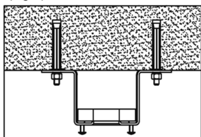
1-SOPORTE MONTAJE
