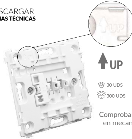
S40.502.00 CONMUTADOR MECANISMO
